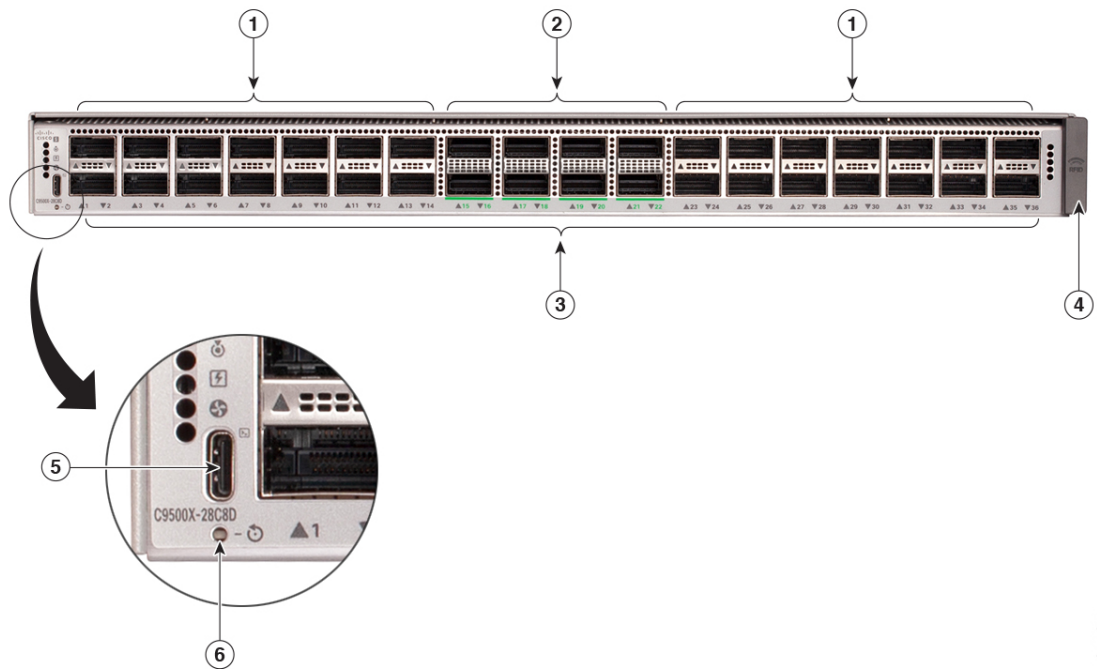
図 1: C9500X-28C8D の前面パネル
