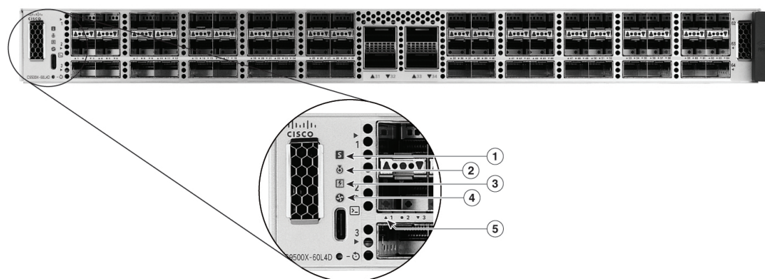
図 49 : C9500X-60L4D の前面パネルの LED
