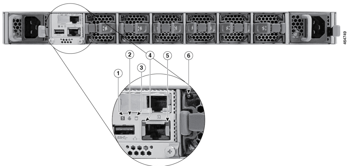
図 50: 背面パネルの LED
