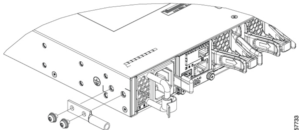
図 11: アースブラケットを使用しないラグの取り付け
