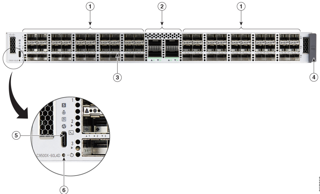
図 2: C9500X-60L4D の前面パネル
