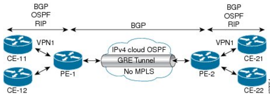
図 1: PE-to-PE トンネリング
