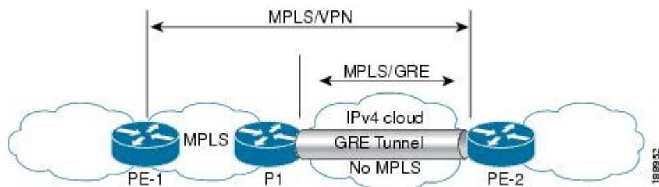
図 2: P-to-PE トンネリング
