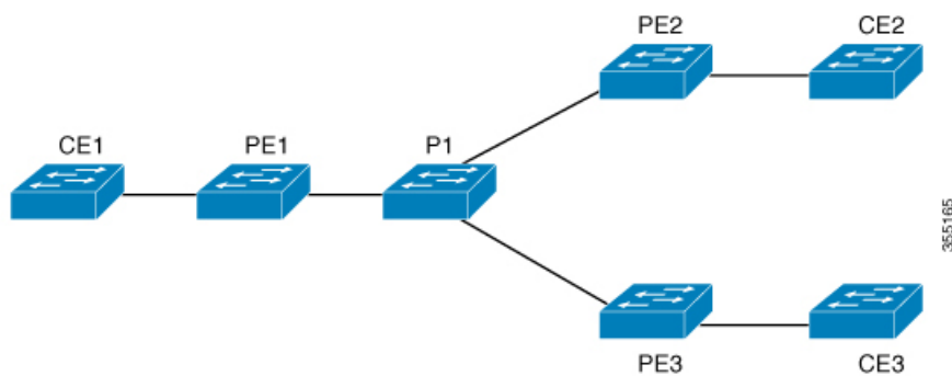
図 1: 6VPE トポロジ
