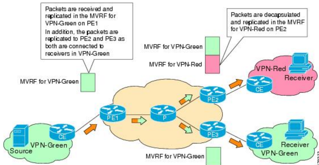
図 2: mVPN エクストラネットサポート設定オプション1の packets フロー
