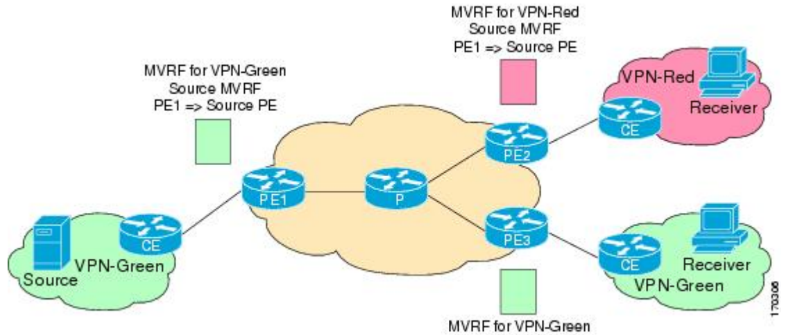
図 1: mVPN エクストラネットのコンポーネント
