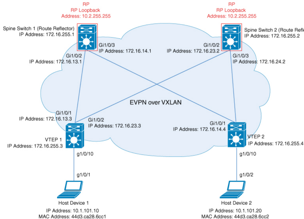
図 4: マルチキャスト レプリケーションによるレイヤ2 VNI を使用した EVPN VXLAN ネットワーク
