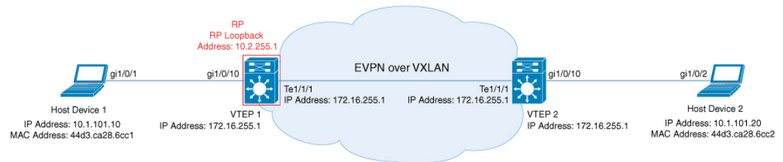
図 2: マルチキャスト複製を使用したレイヤ2 VNI を備えた EVPN VXLAN ネットワーク
