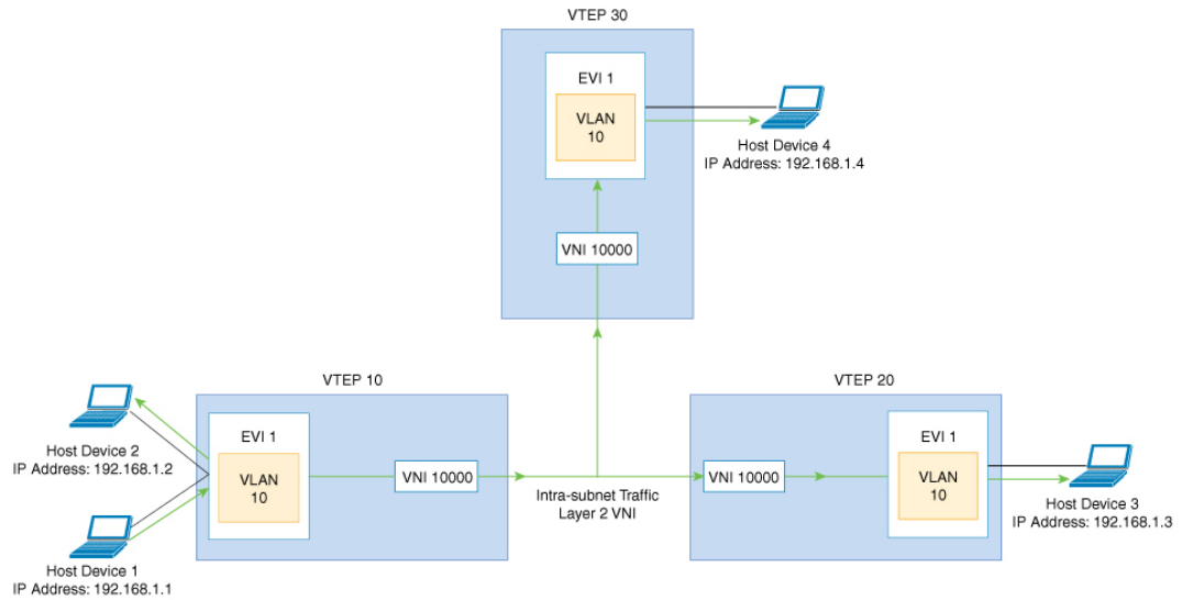
図 1: レイヤ2 VNI を介した BUM トラフィック
