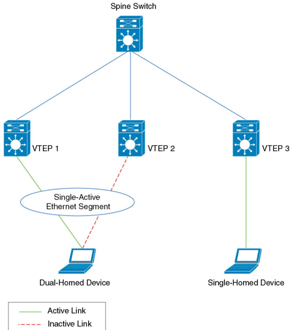
図 2: デュアルホーム接続デバイスのトポロジ
