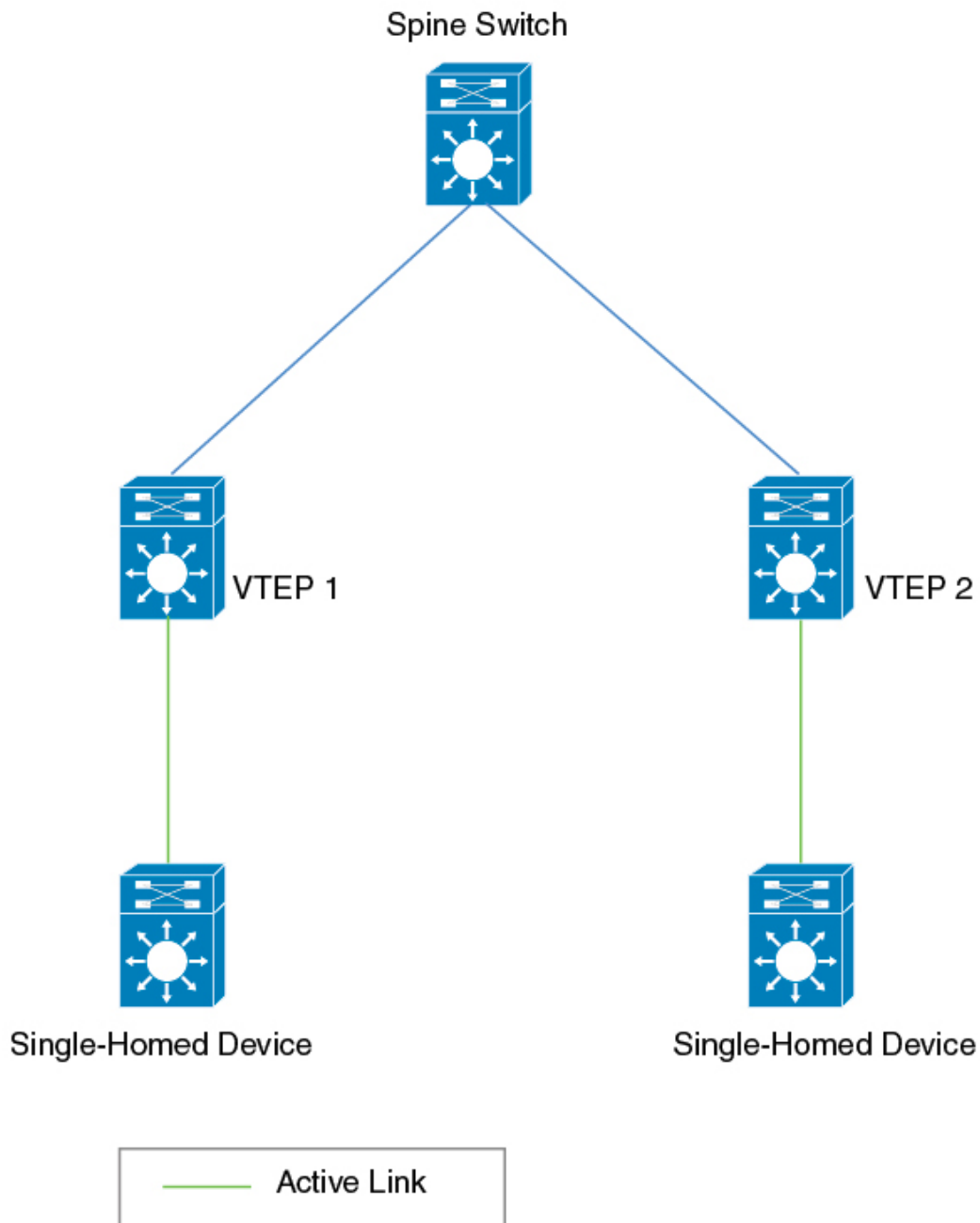
図 1: シングルホームのトポロジ
