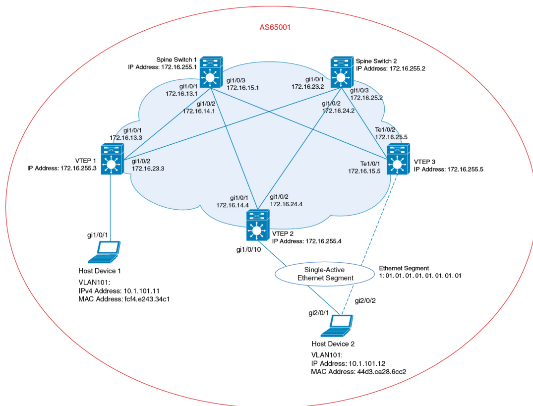
図 6: BGP EVPN VXLAN ファブリック内でのシングルアクティブ冗長性を備えたデュアルホーミングの設定
