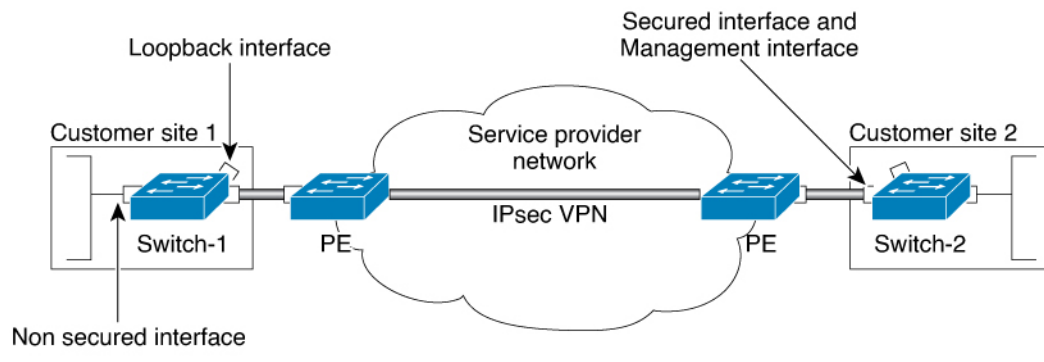
図 44：IPsec ネットワーク
