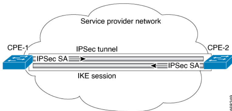
図 45: IPsec トンネル
