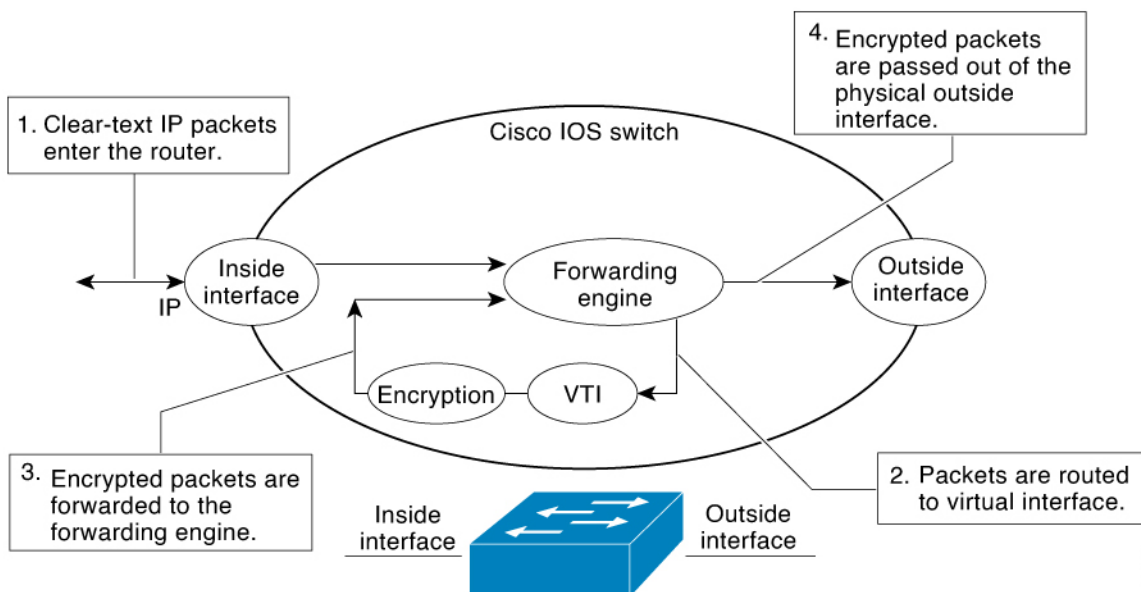
図 47: IPsec トンネルへのパケットフロー
