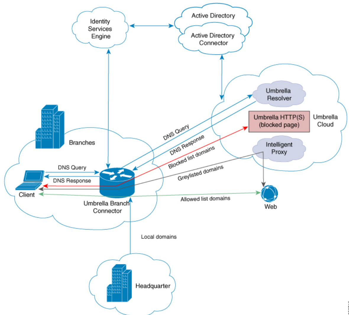
図 50: Cisco Umbrella 統合を使用したクラウドベースのセキュリティサービス (Cisco Identity Services Engine と Umbrella Active Directory コネクタを使用)
