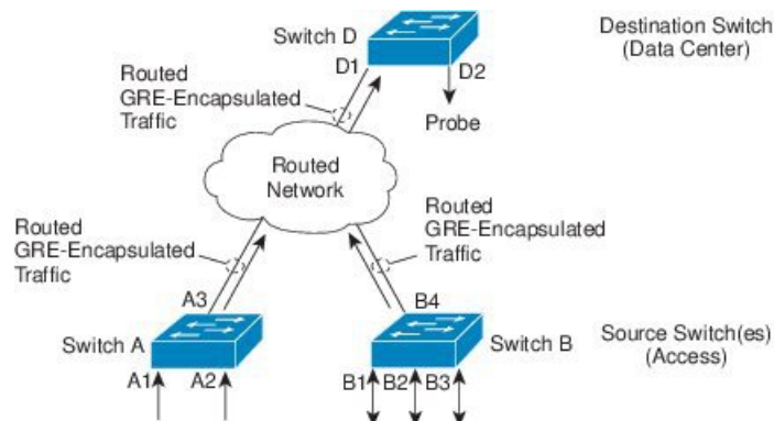
図 9: ERSPAN の設定
