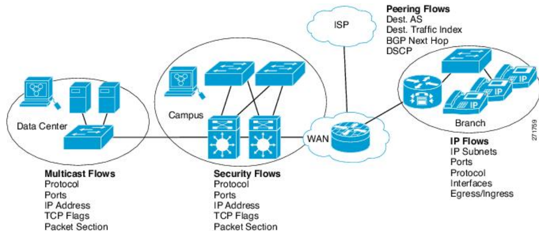
図 10: Flexible NetFlow の通常の導入
