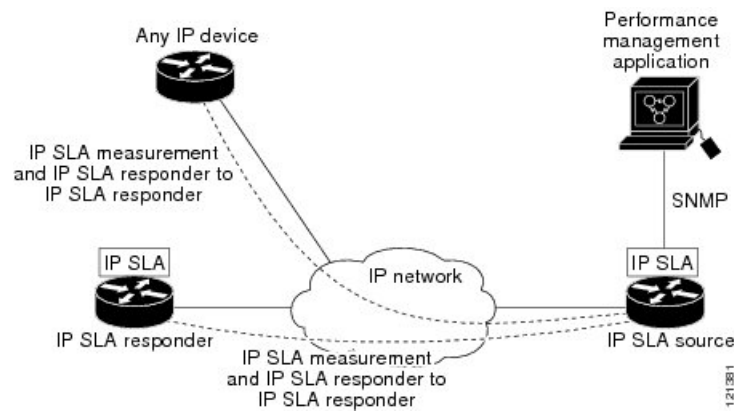
図 4: Cisco IOS IP SLA 動作
