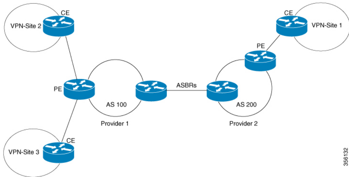
図 9: Redistribute Connected Subnet 方式を使用した InterAS オプション B のトポロジ
