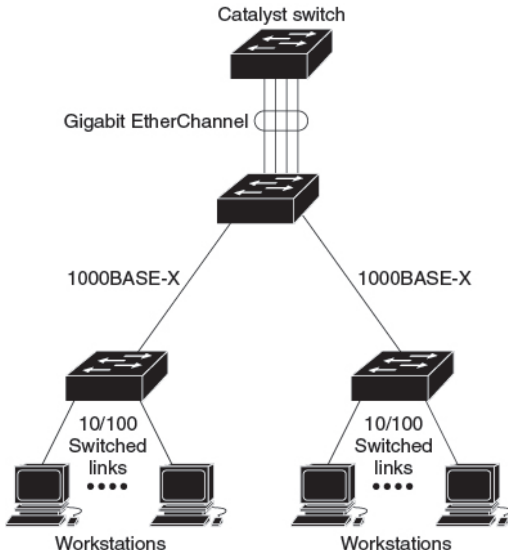
図 1: 一般的な EtherChannel 構成
