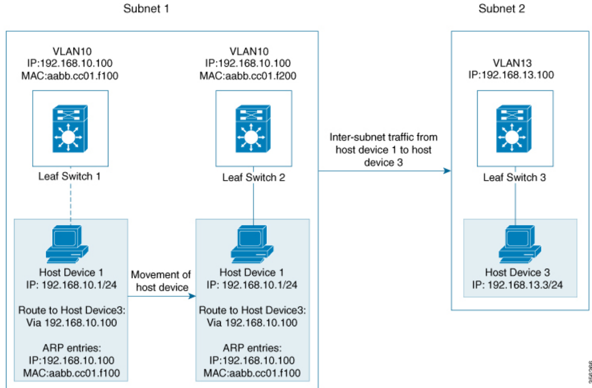
図 5:分散型ゲートウェイポロジ
