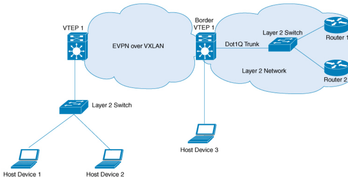
図 29: IEEE 802.1Q ネットワークとのレイヤ 2 外部接続
