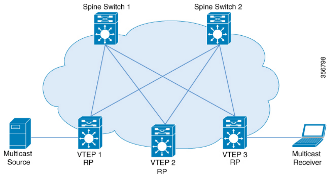
図 15: オーバーレイネットワークのエニーキャスト RP
