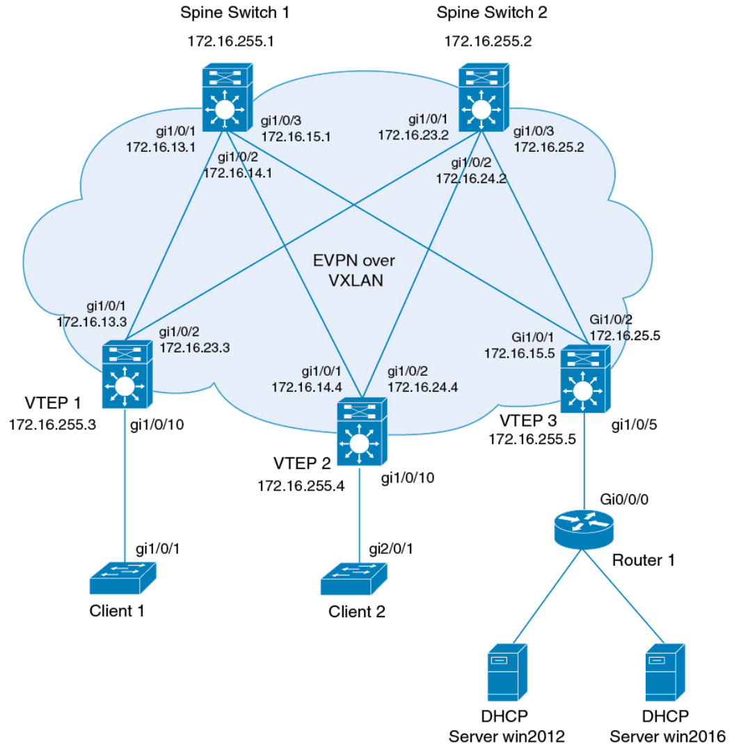
図 12: BGP EVPN VXLAN ファブリック内での DHCP リレーの展開
