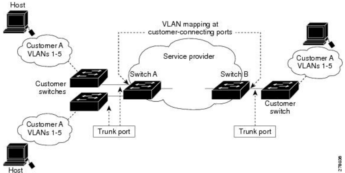
図 1: カスタマー VLAN からサービスプロバイダー VLAN へのマッピング
