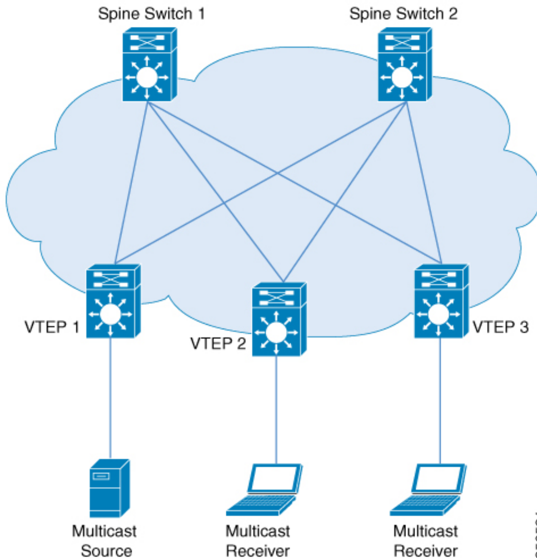
図 14: テナントルーテッドマルチキャストトポロジ
