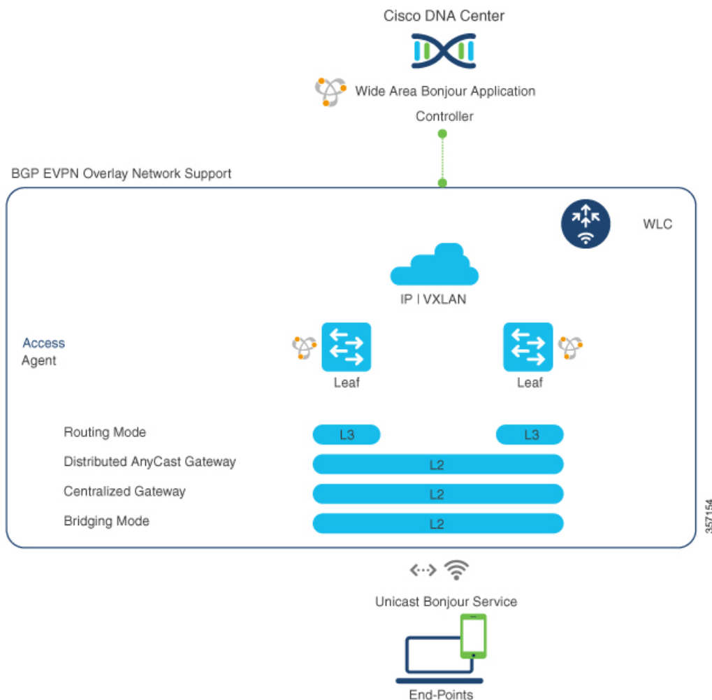
図 43: BGP EVPN 対応エンタープライズ ネットワークのオーバーレイ Bonjour サービス
