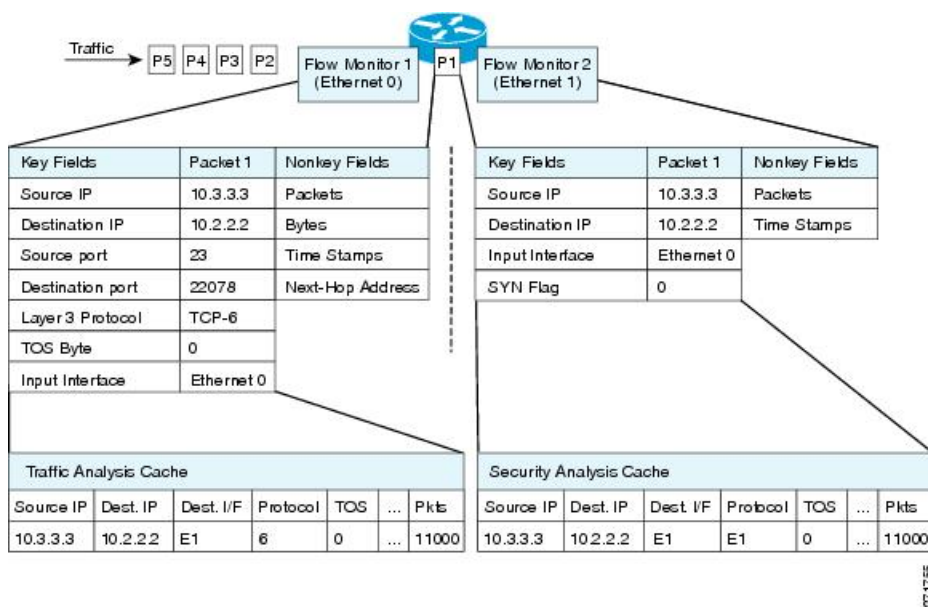
図 12:2 つのフロー モニターを使用した同じトラフィックの分析例
