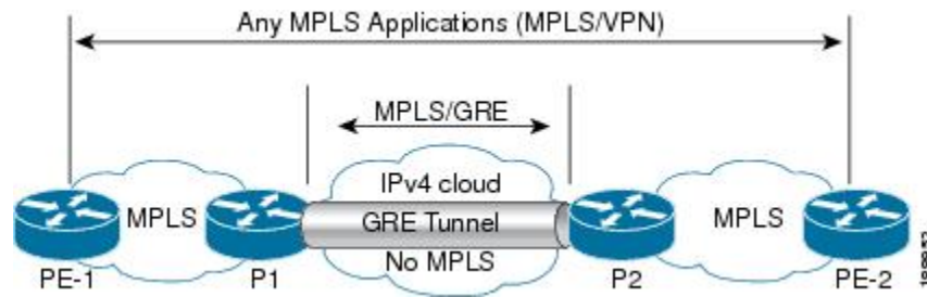
図 12: P-to-P トンネリング
