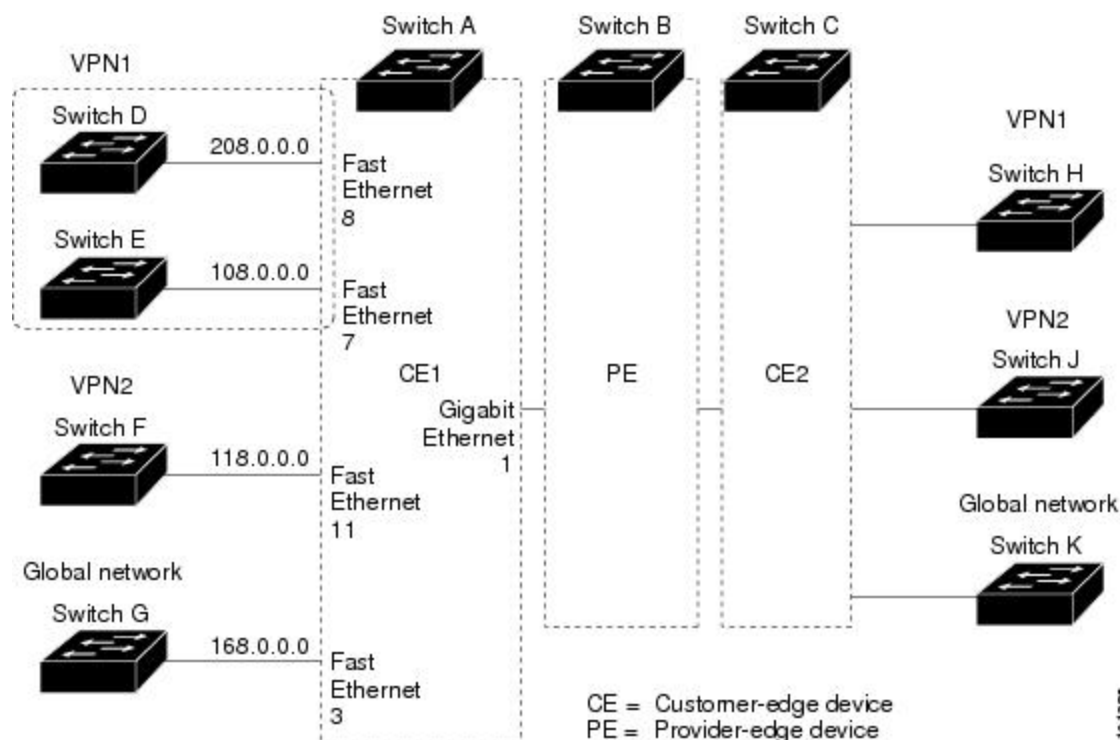
図 14: Multi-VRF CE の設定例
