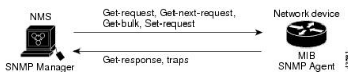
図 1: SNMP ネットワーク
