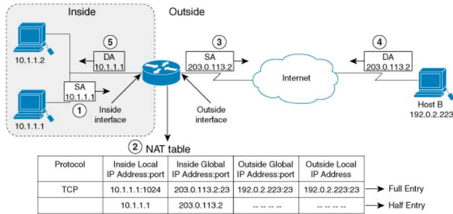
図 16: NAT 内部送信元変換
