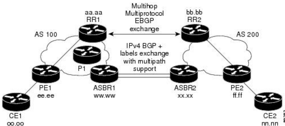
図 26: IPv4 ルートおよび MPLS ラベルを交換する 2 つの VPN サービス プロバイダーの設定
