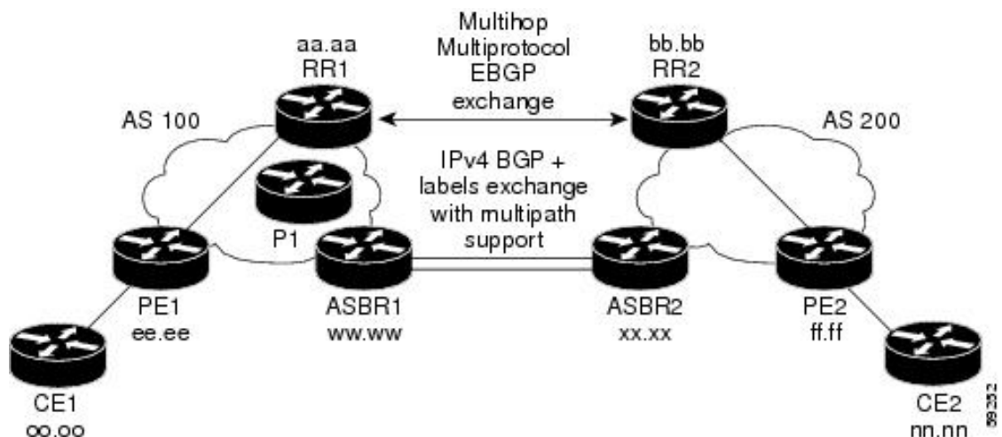
図 27: MPLS VPN サービスプロバイダー間での IPv4 ルートと MPLS ラベルの配布
