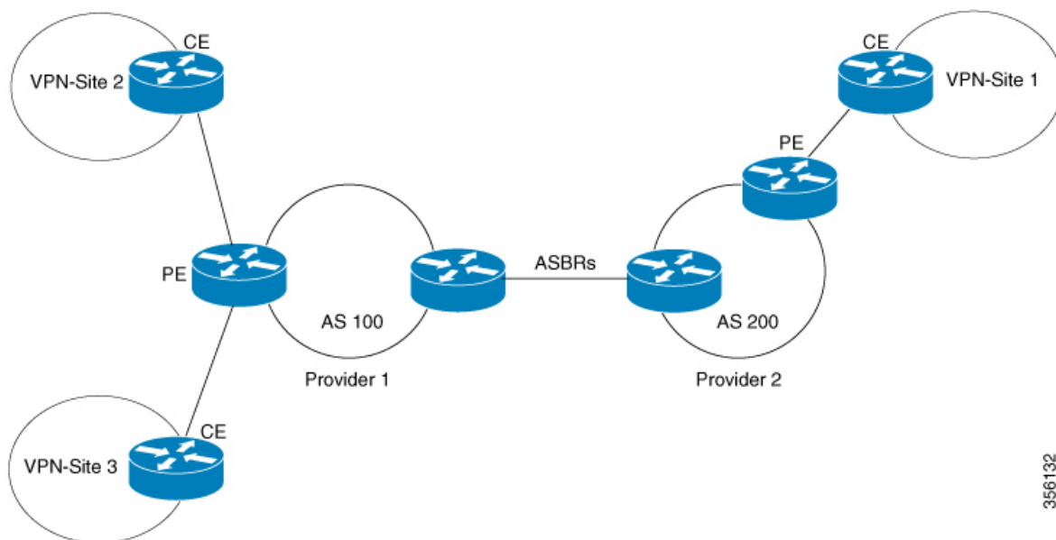
図 8: Redistribute Connected Subnet 方式を使用した InterAS オプション B のトポロジ
