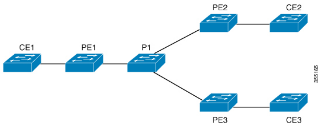
図 23: 単一の MPLS VPN 自律システム トポロジのプロバイダー エッジ (PE) デバイスでのルート ターゲットの置換
