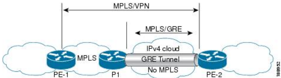
図 19: P-to-PE トンネリング
