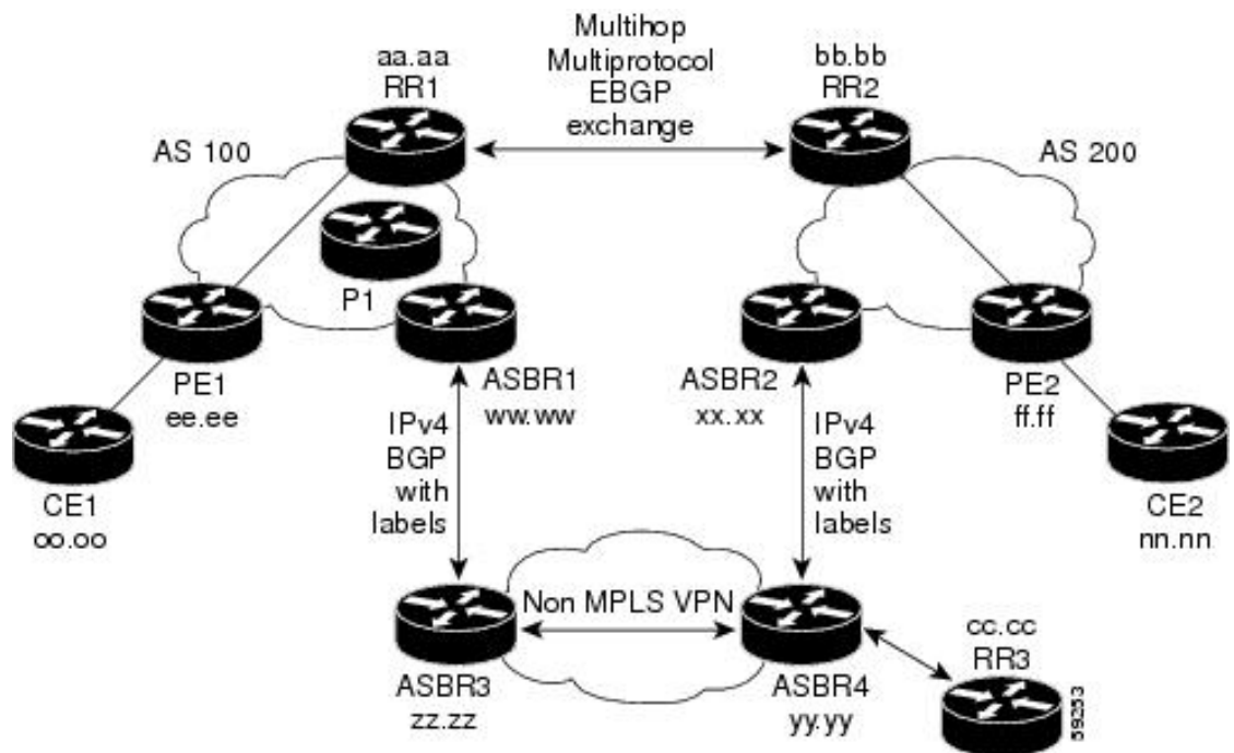
図 28: 非 MPLS VPN サービスプロバイダー経由でのルートと MPLS ラベルの配布
