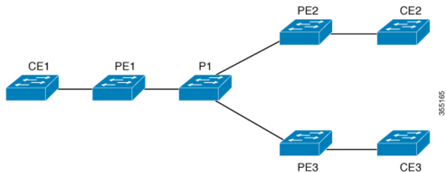
図 22: VPLS トポロジ
