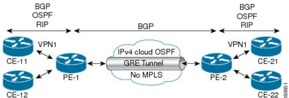
図 18: PE-to-PE トンネリング
