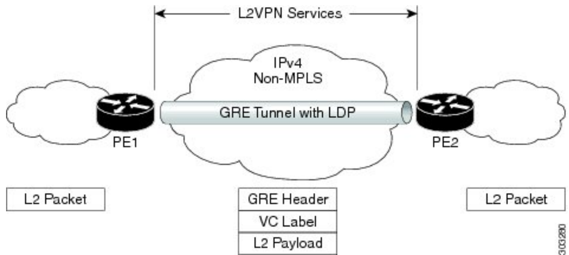
図 15: PE-to-PE トンネリング
