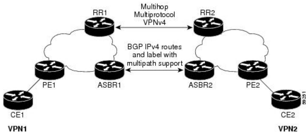
図 24: EBGP および IBGP を使用してルートと MPLS ラベルを配布する VPN
