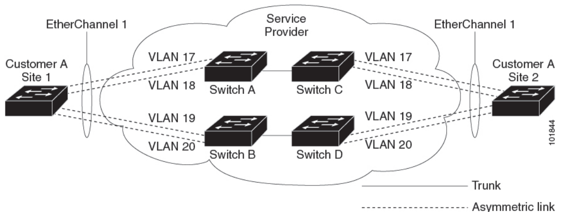
図 31: EtherChannel のレイヤ2 プロトコル トネリング
