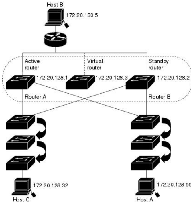
図 11: HSRP の一般的な構成
