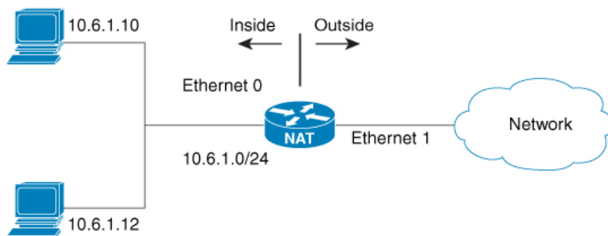
図 15: NAT
