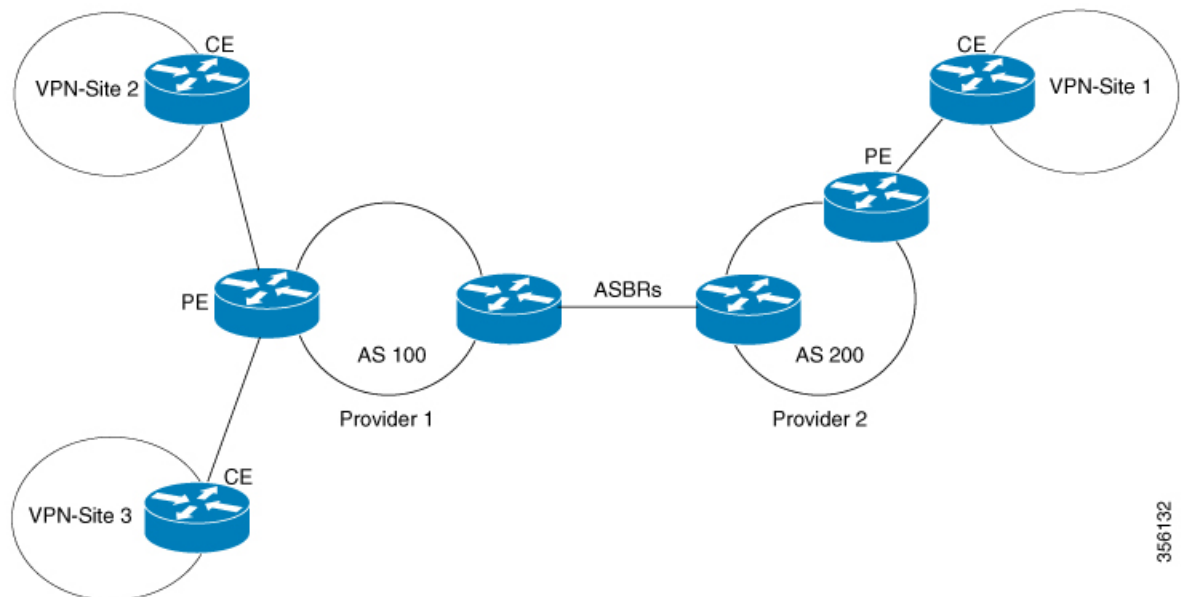
図 2: Redistribute Connected Subnet 方式を使用した InterAS オプション B のトポロジ
