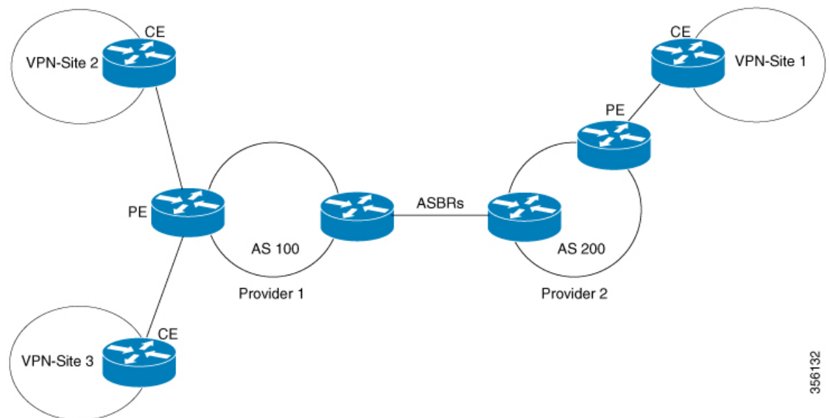
図 1: ネクストホップセルフ方式を使用した InterAS オプション B のトポロジ
