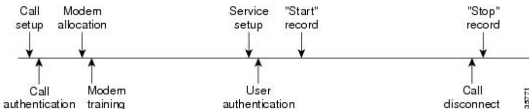
図4:通常のフローでAAAリソース失敗終了アカウントティングを有効にしていないモデムダイヤルインコール設定シーケンス
