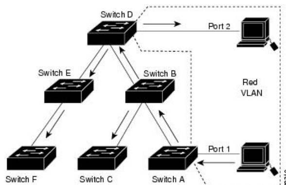
図 2: VTP プルーニングによるフラディングトラフィックの最適化
