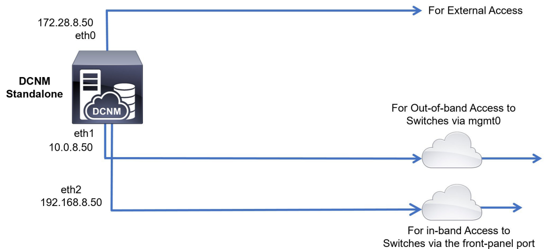
図 3: コンピューティング クラスタを使用しない Cisco DCNM スタンドアロン展開
