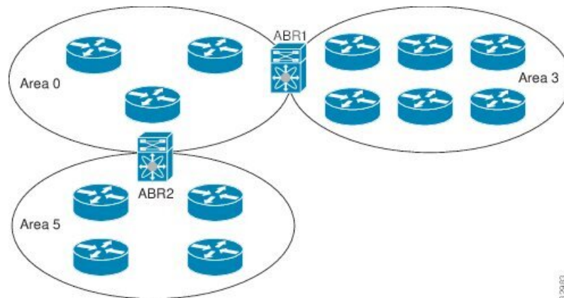
図 21: OSPFv3 エリア
