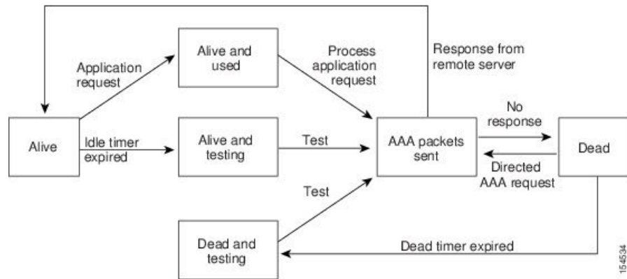
図 1: LDAP ????????
