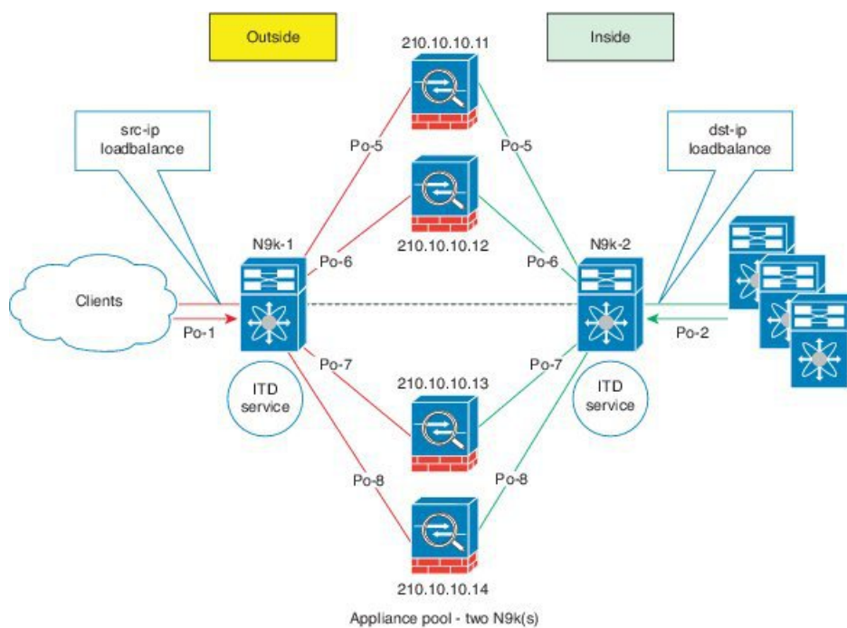
図 15: サンドイッチ展開モード
