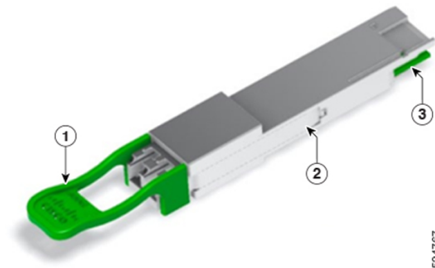
図 5: 800 ギガビット QSFP-DD トランシーバモジュール
