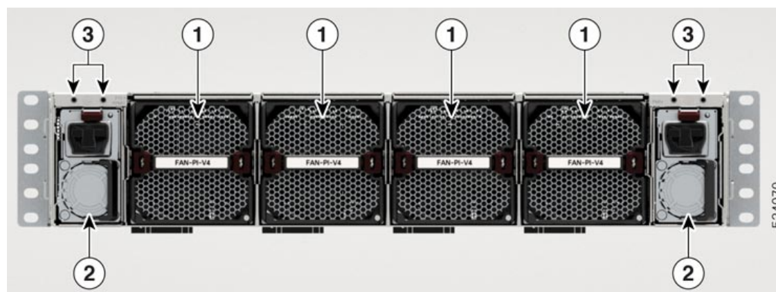
図 2: Cisco Nexus 9364E-SG2-Q スイッチ：背面図
