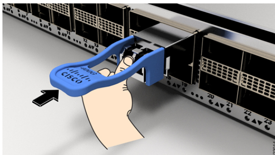
図 7: QSFP トランシーバモジュールの装着
