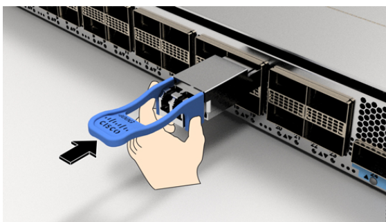
図 6: QSFP トランシーバモジュールの取り付け
