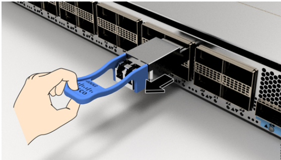
図 9: QSFP トランシーバモジュールの取り外し
