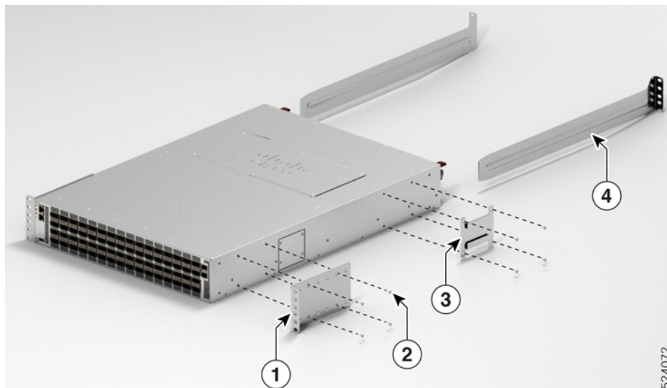
図 4: Cisco Nexus N9364E-SG2-Q スイッチのラック マウント ブラケット : ポート側吸気
