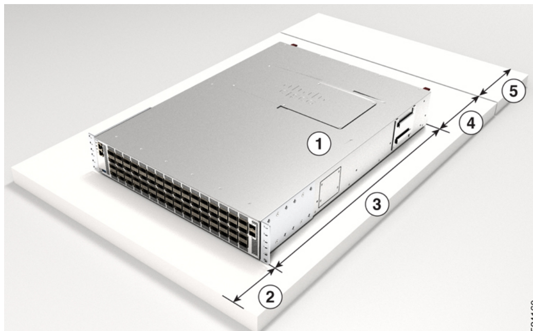
図 3: Cisco Nexus N9364E-SG2-Q のシャーシ周囲に必要なスペース
