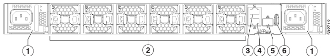
図 2: Cisco Nexus 9316D-GXスイッチの電源側面図
