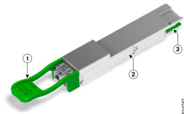
図 2: 800 ギガビット QSFP-DD トランシーバモジュール
