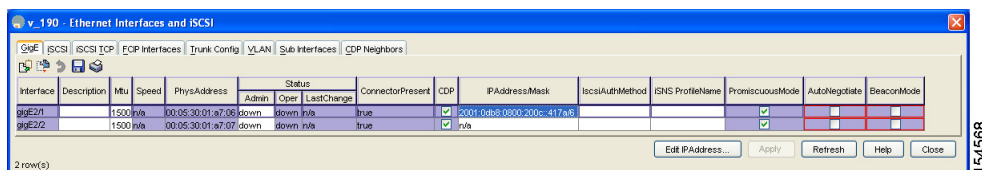
図 8-11 Device Manager の [Gigabit Ethernet Configuration] ダイアログボックス
