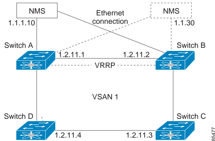
図 5-10 VRRP の機能
