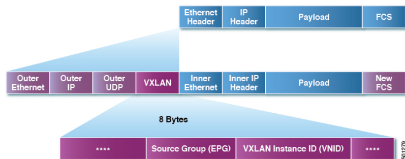
図 41: ACI VXLAN のパケット形式
