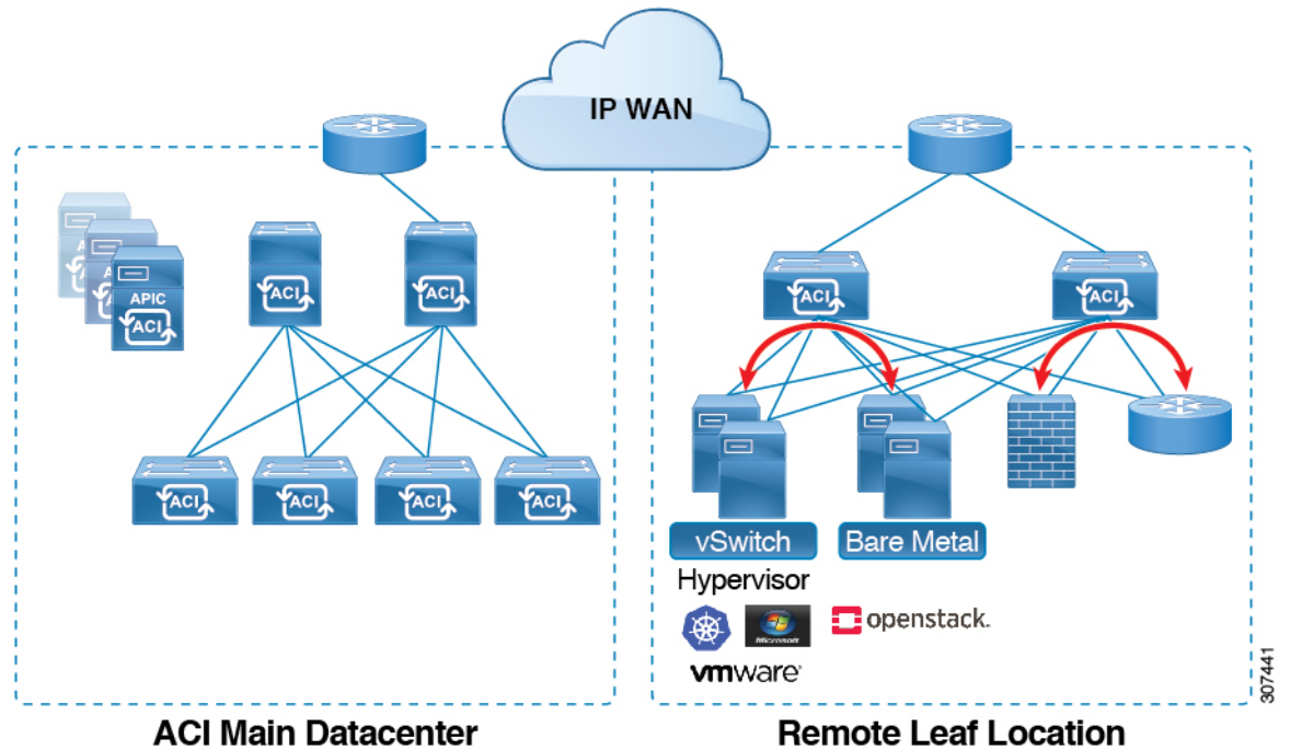
図 78 : Local Switching Traffic : リリース 4.1(2) 以前
