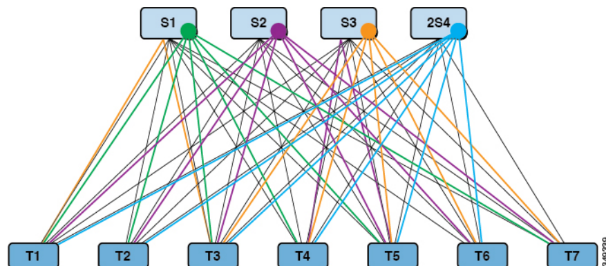
図 48: マルチキャスト ツリー トポロジ
