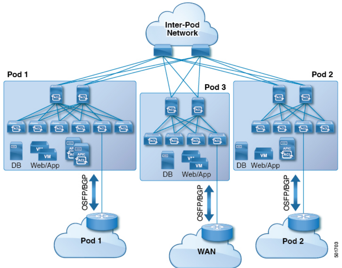
図 88: 中継ルーティング設定における L3Out を伴う複数のポッド
