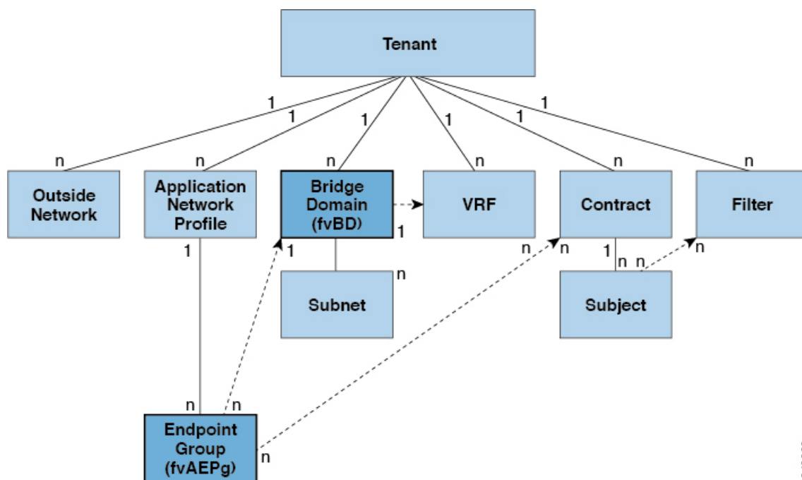
図 20: MO の関係
