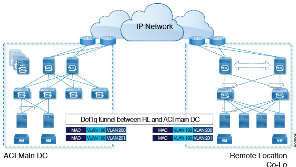
図 82: リモートリーフスイッチの動作、リリース 4.2 (4) : リモートリーフスイッチでの 802.1Q トンネルサポート
