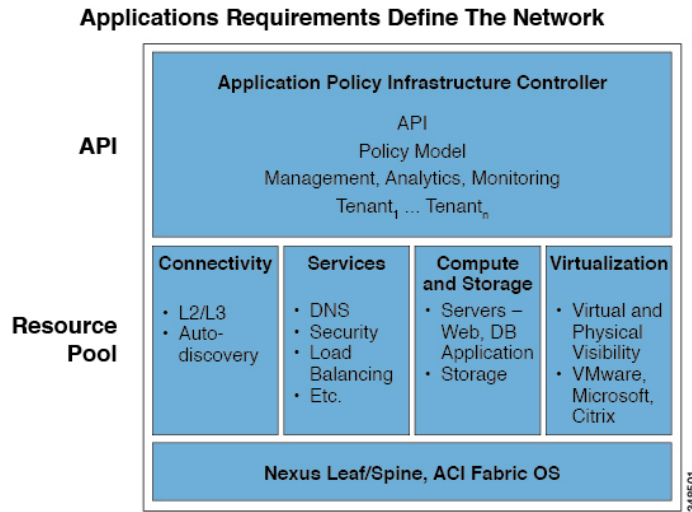
図 1: APIC の概要
