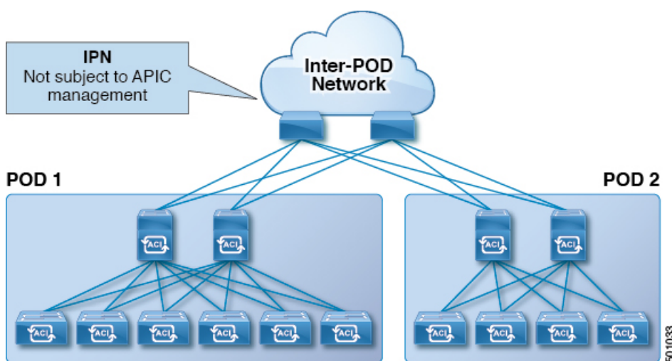
図 77: マルチポッド トポロジ
