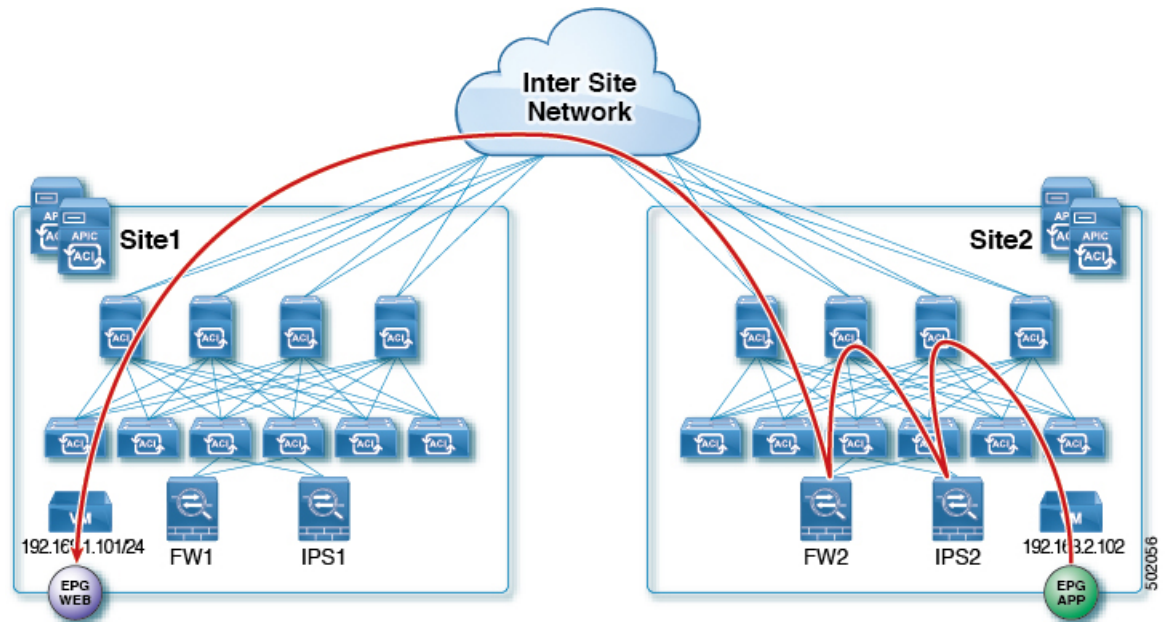
図 13: イーストウェスト FW/IPS リバーストラフィック
