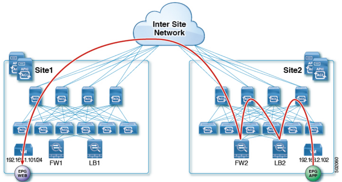
図 15: イーストウェスト FW/LB リバーストラフィック
