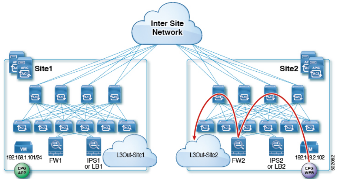
図 7: ノースサウス FW リバーストラフィック
