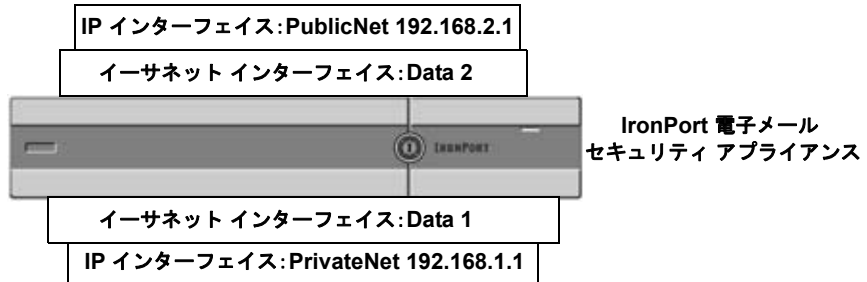
図 3-15 パブリック インターフェイスとプライベート インターフェイスの例
