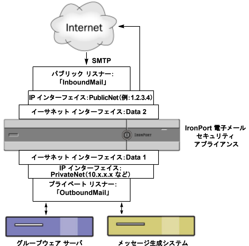
図 2-1 エンタープライズ ゲートウェイ設定のパブリック リスナーおよびプライベート リスナー
