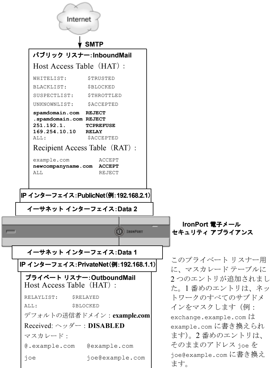
図 3-5 プライベート リスナー用に定義されたマスカレード
