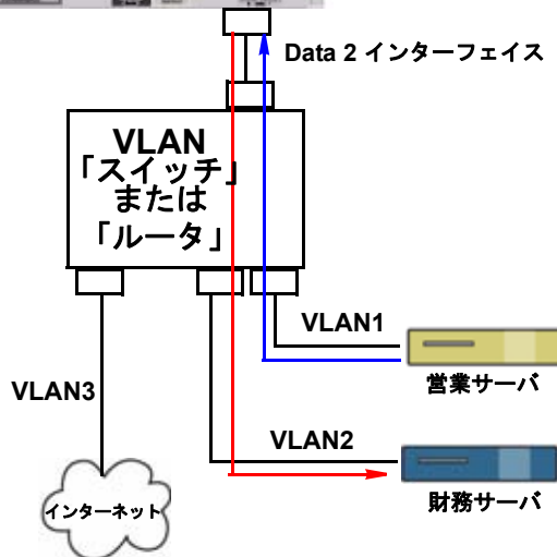
図 7-2 VLAN によるアプライアンス間通信の実現 VLAN1、VLAN2、VLAN3 用に 設定された IronPort アプライアンス
