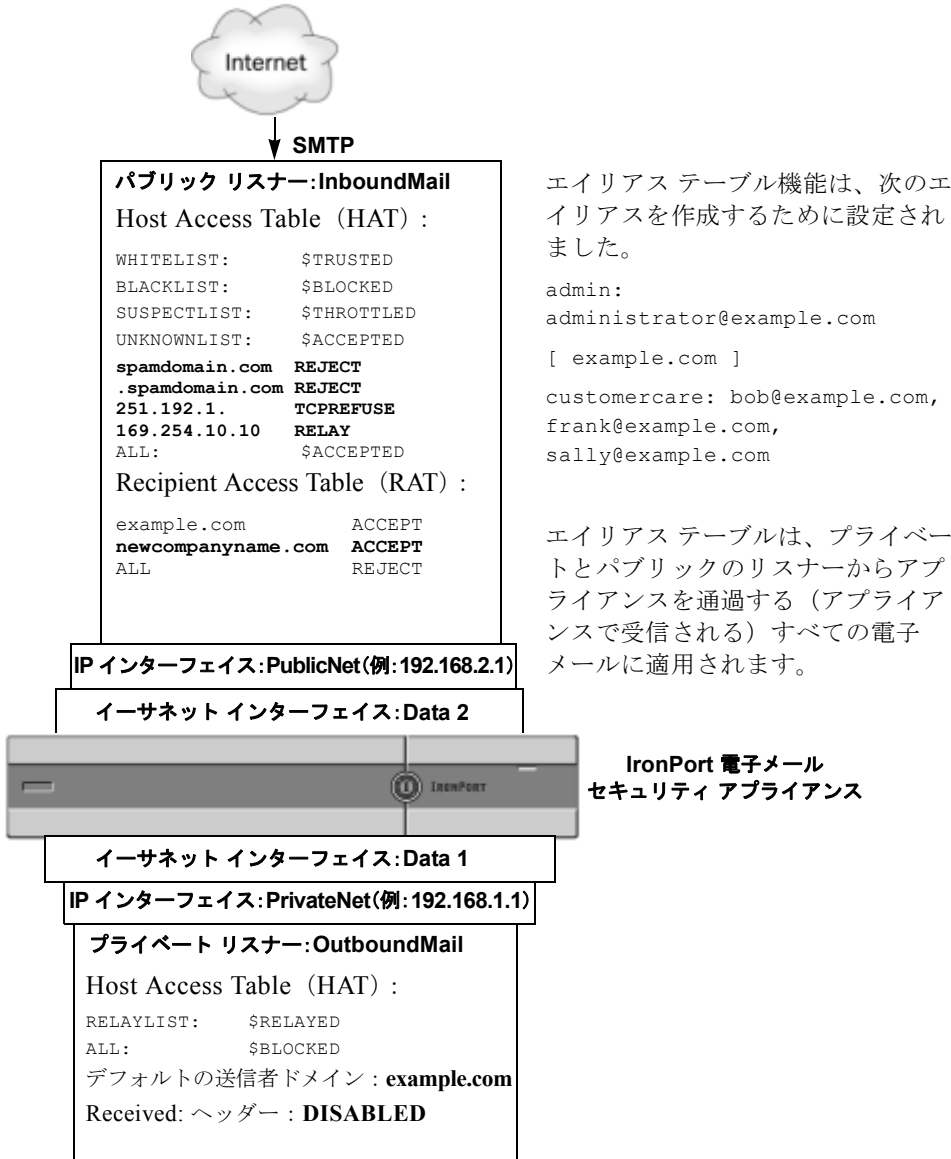
図 3-4 アプライアンスに定義されたエイリアス テーブル
