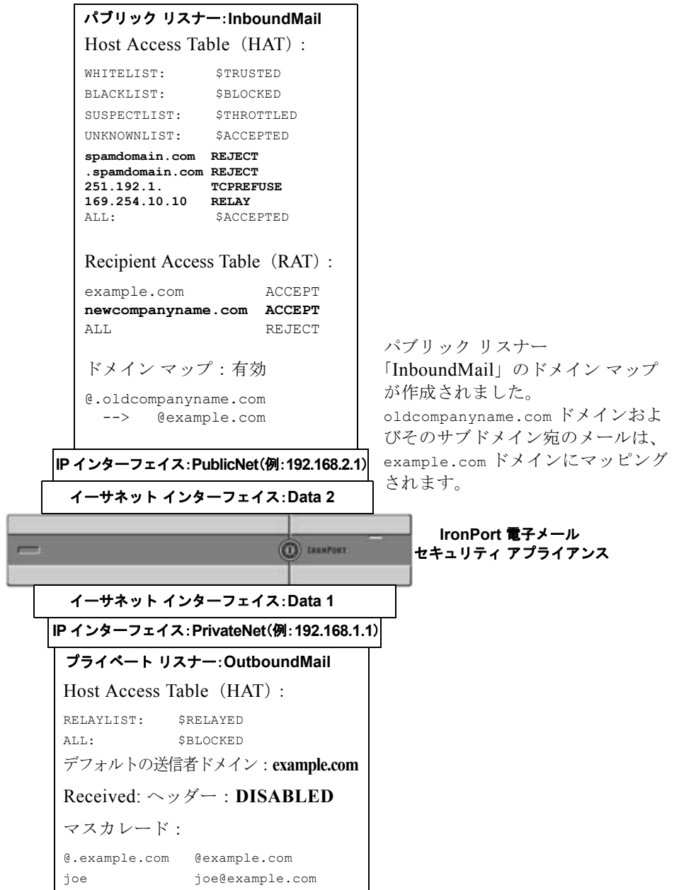
図 3-6 パブリック リスナー用に定義されたドメイン マップ
