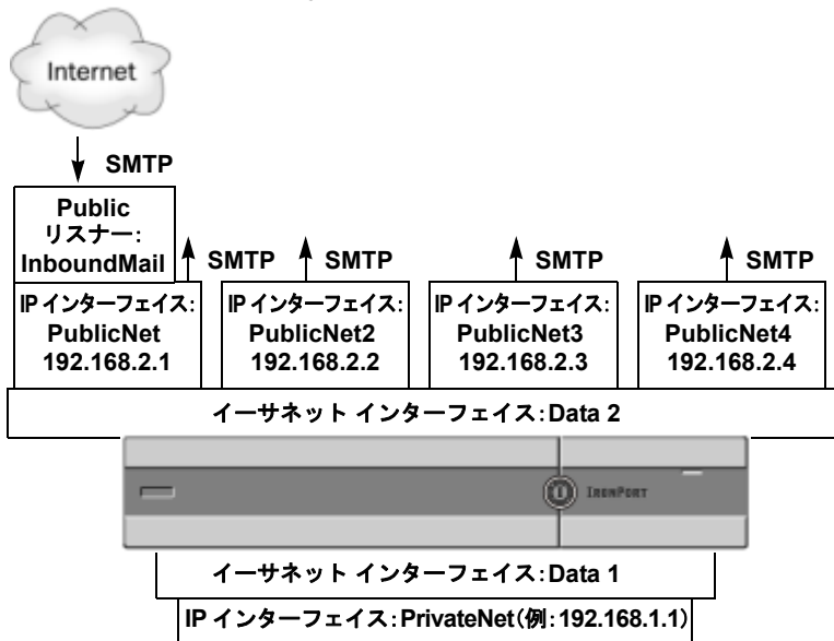
図 3-19 1 つのイーサネット インターフェイス上にある 4 つの Virtual Gateway アドレス
