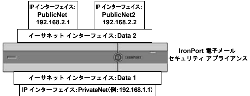
図 3-18 別のパブリック インターフェイスの追加
