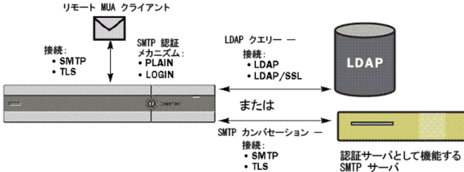
図 4-16 SMTP Auth のサポート : LDAP ディレクトリ ストアまたは SMTP サーバ
