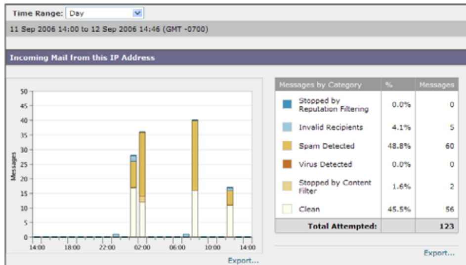
図 2-12 IP アドレス プロファイル ページ (1/2)
