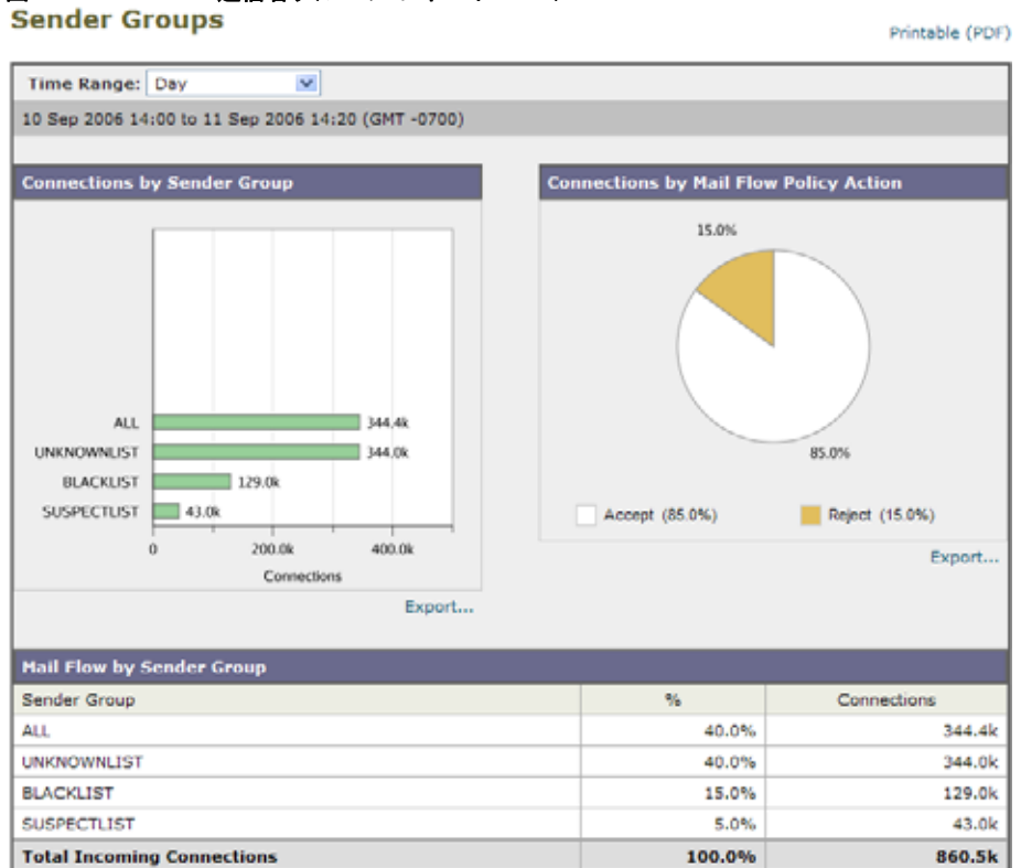
図 2-14 送信者グループ レポート ページ
