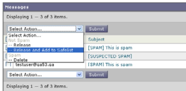
図 4-28 エンドユーザ検疫内のセーフリスト
