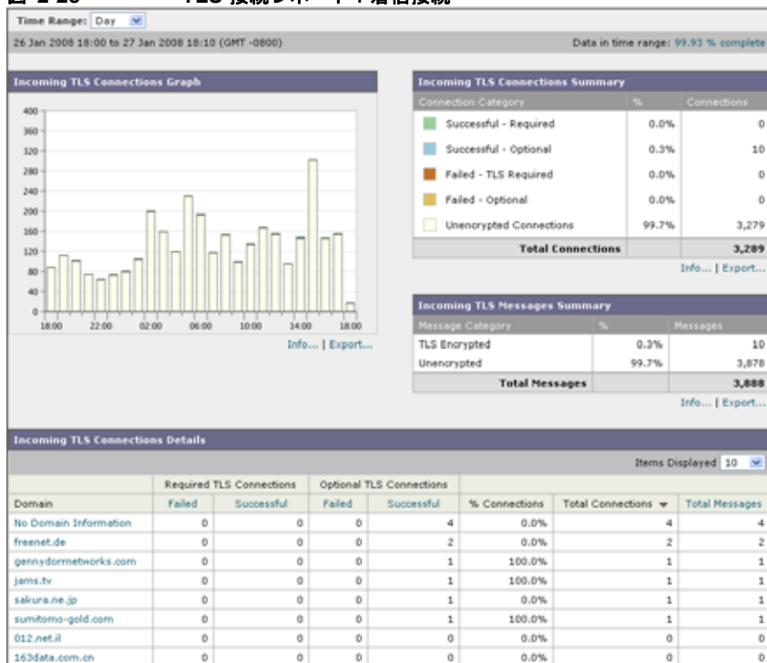
図 2-28 TLS 接続レポート：着信接続
