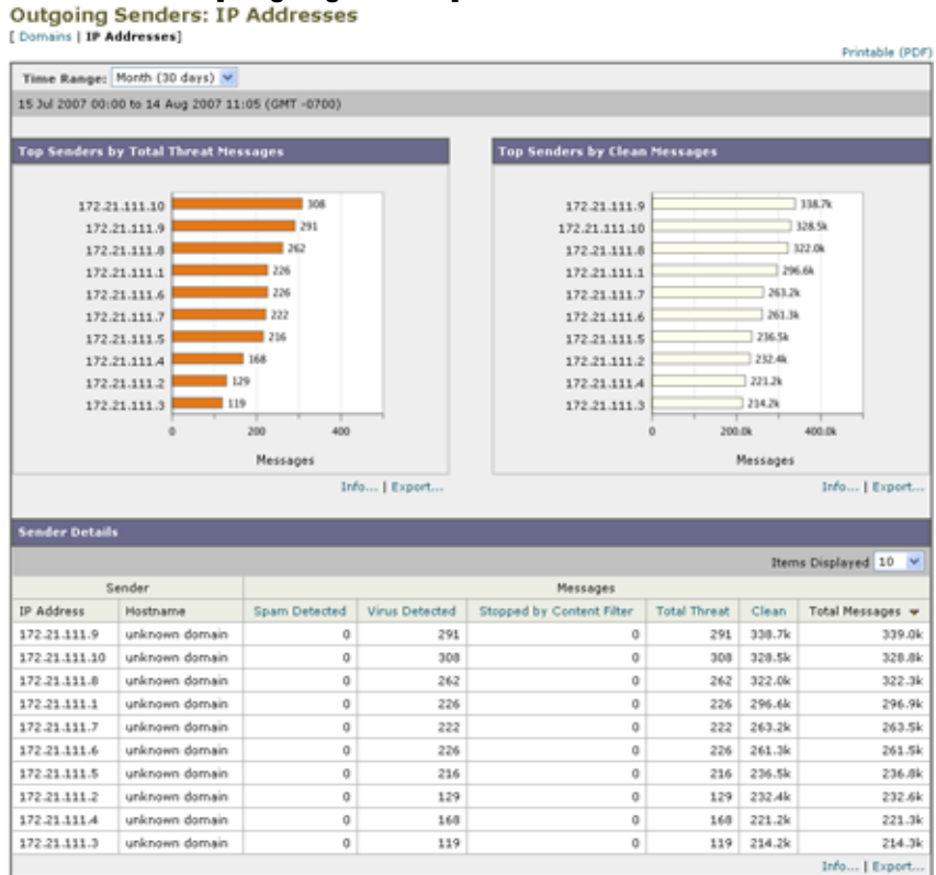
図 2-16 [Outgoing Senders] ページ (IP アドレスを表示中)
