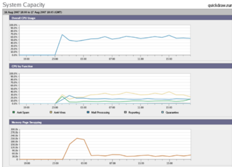
図 2-36 [System Capacity] : [System Load] (高負荷時のシステム)
