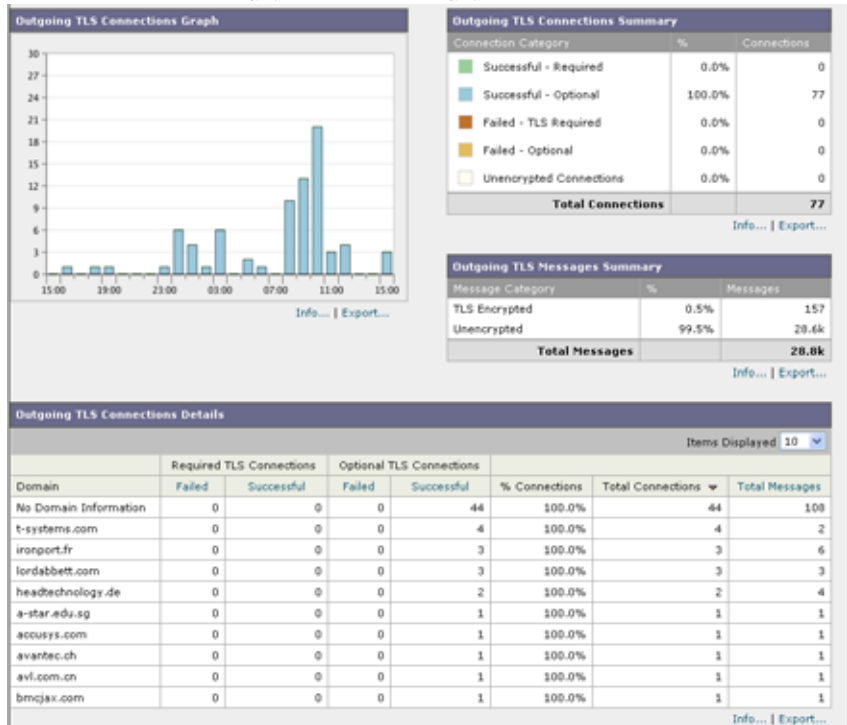
図 2-29 TLS 接続レポート：発信接続
