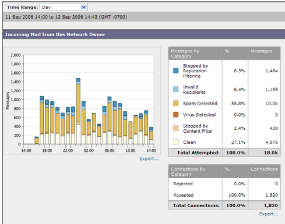
図 2-10 ネットワーク オーナー プロファイル ページ (1/2)
