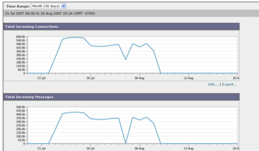
図 2-31 [System Capacity] : [Incoming Mail] (1/2 ページ)
