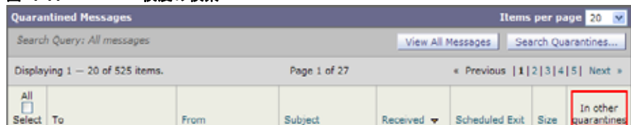
図 4-11 検疫の検索
