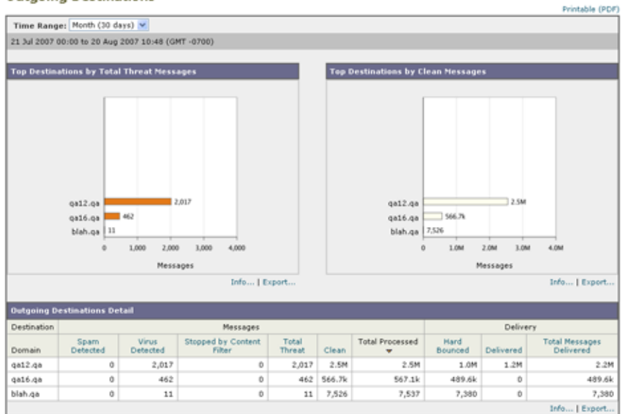
図 2-15 [Outgoing Destinations] ページ Outgoing Destinations
