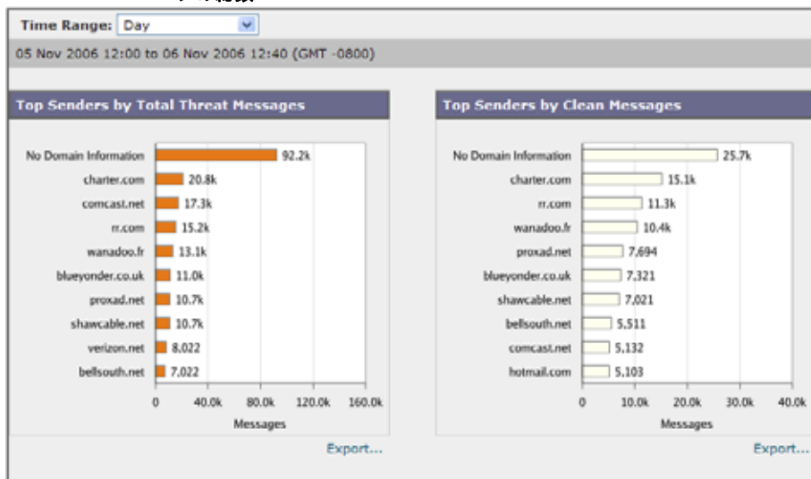
図 2-4 着信メールのグラフ：脅威メッセージの総数およびクリーン メッセージの総数
