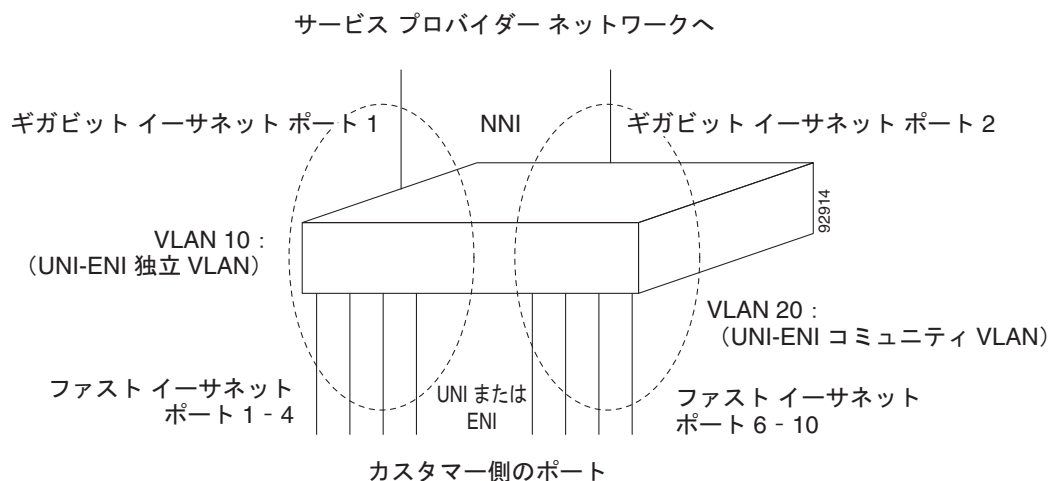
図 12-2 Cisco ME スイッチの UNI-ENI 独立 VLAN および UNI コミュニティ VLAN
