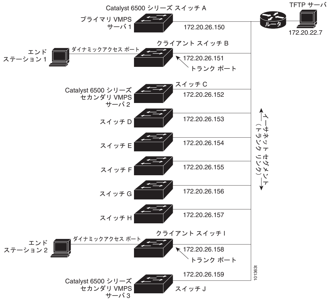
図 12-5 ダイナミック ポート VLAN メンバーシップの構成
