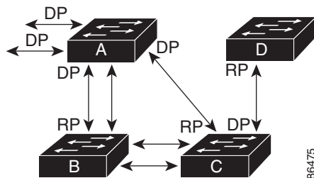
図 15-2 スパニング ツリー トポロジ
