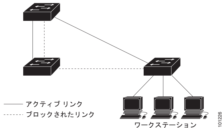
図 15-3 スパンニング ツリーおよび冗長接続
