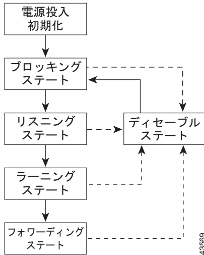
図 15-1 スパニング ツリー インターフェイスのステート
