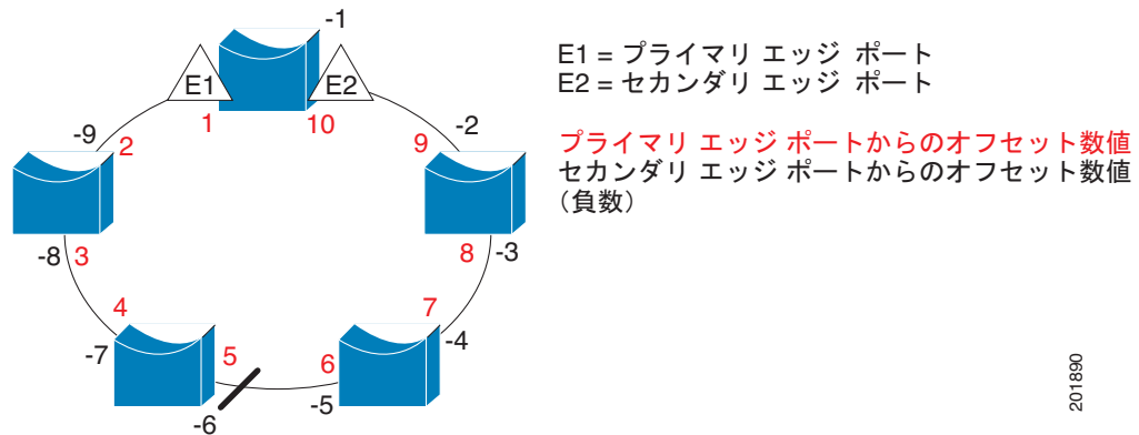
図 18-4 セグメント内のネイバー オフセット番号
