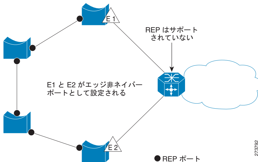
図 18-3 エッジ非ネイバー ポート
