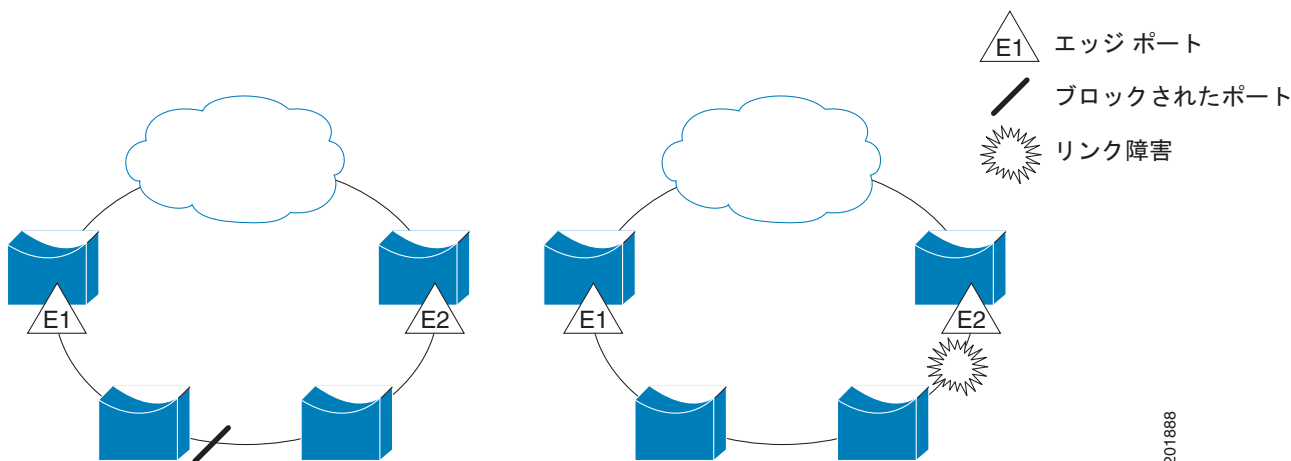
図 18-1 REP オープン セグメント
