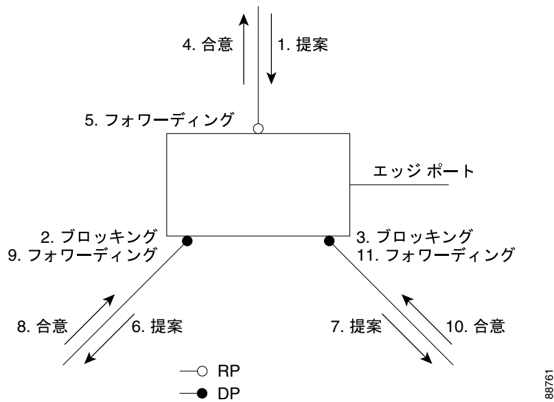
図 18-5 高速コンバージェンス中のイベント シーケンス
