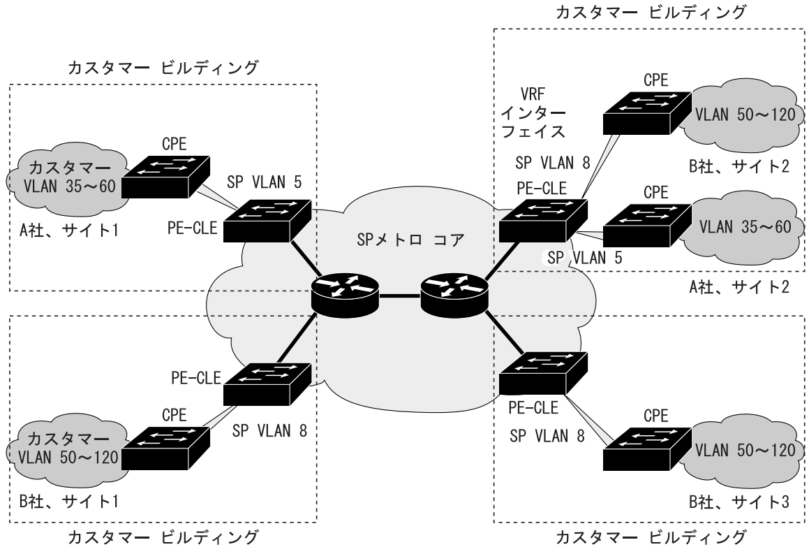
図 1-2 レイヤ2 VPN 構成
