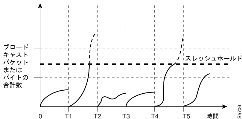
図 34-1 ブロードキャスト抑制
