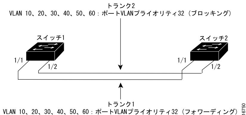
図 5-3 VLAN トラフィック負荷分散設定前の並列トランク設定
