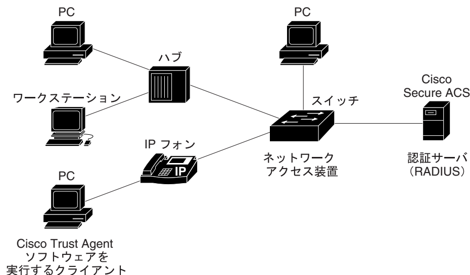
図 46-2 NAC レイヤ 2 IP を使用するネットワーク
