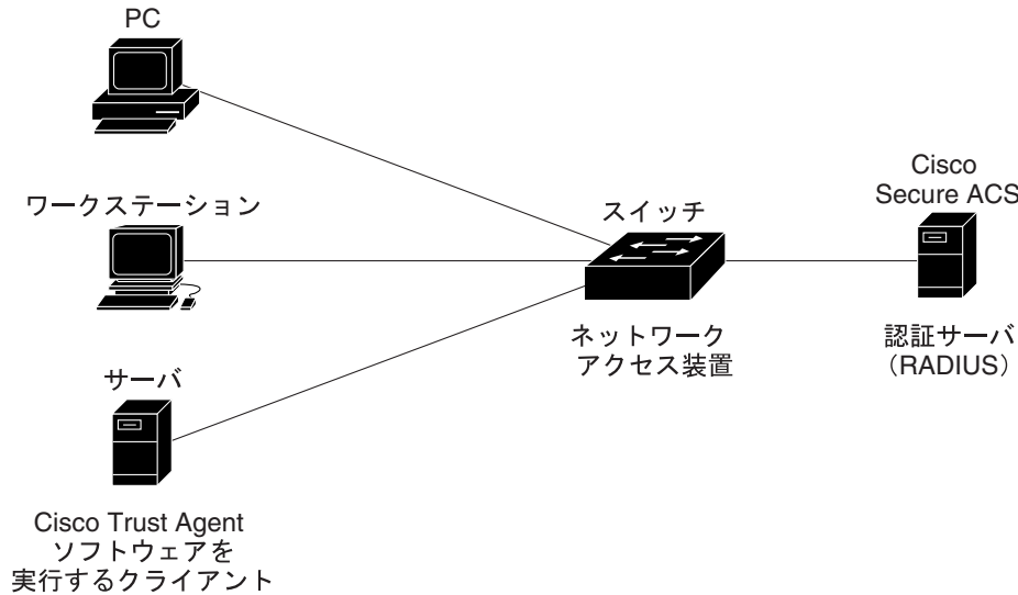
図 46-1 ポスチャ検証装置
