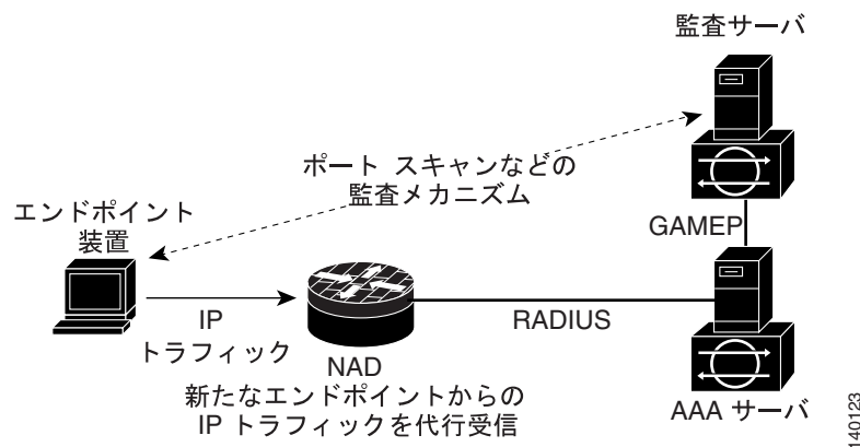
図 46-3 NAC 装置の役割
