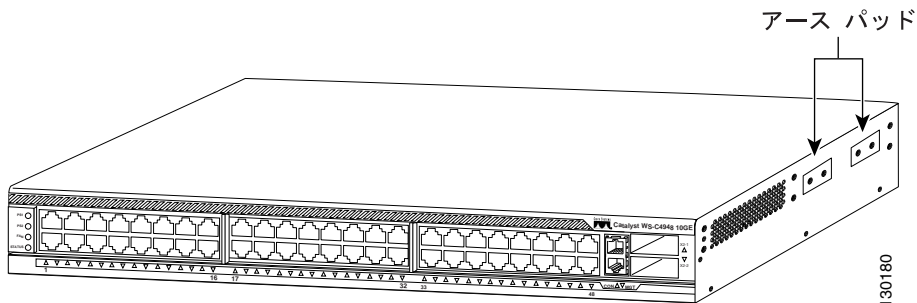
図 2-1 アースパッドの位置
