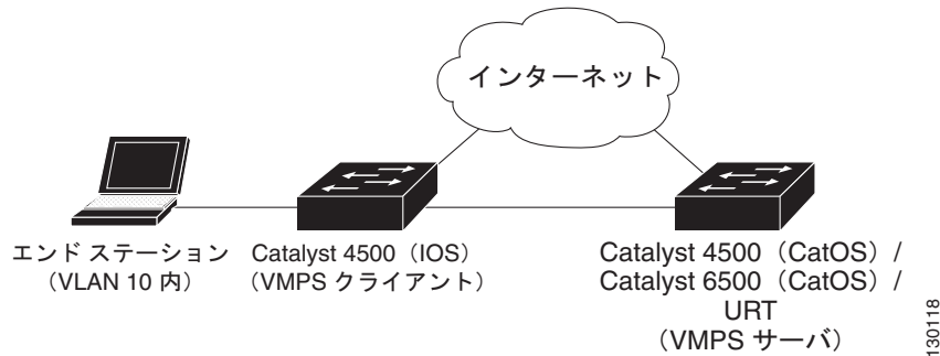
図 15-5 ダイナミックポート VLAN メンバーシップの構成例
