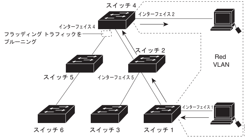
図 15-3 VTP プルーニングを使用した場合のフラッディング Traffic
