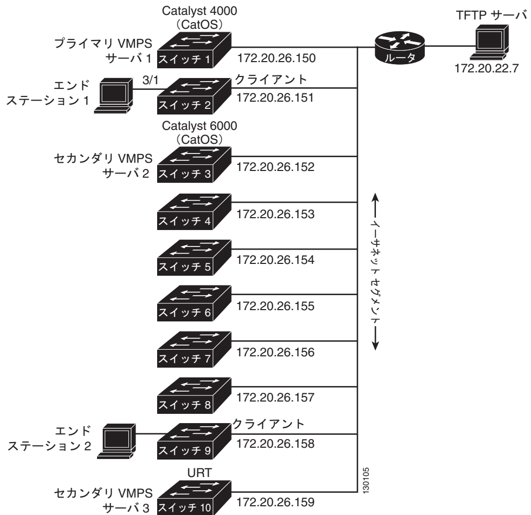
図 15-4 ダイナミック ポート VLAN メンバーシップの構成例
