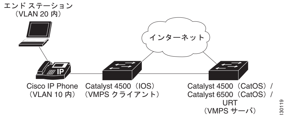
図 15-6 ダイナミックポート VLAN メンバーシップの構成例
