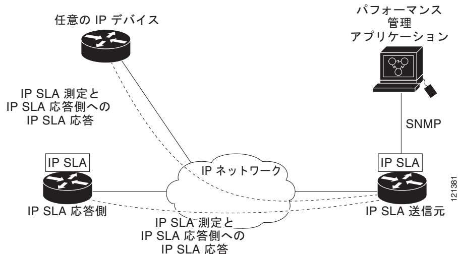
図 66-1 Cisco IOS IP SLA 動作
