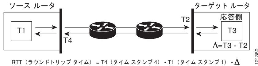
図 66-2 Cisco IOS IP SLA Responder タイムスタンプ
