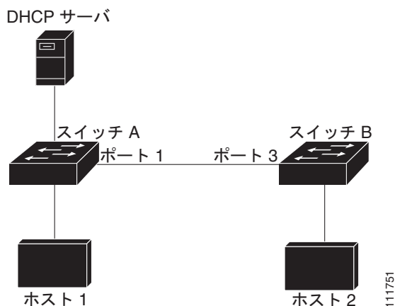
図 39-3 DAI がイネーブルな VLAN 上での ARP パケットの確認
