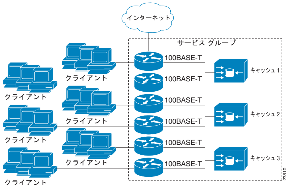
図 60-1 WCCP を使用した Cisco Content Engine ネットワーク構成
